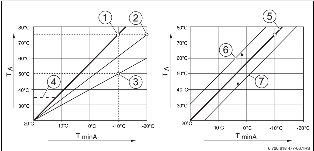
Bild 7 Einstellung der Heizkurve. Links: Einstellung der Steigung über Auslegungstemperatur und minimale Außentemperatur. Rechts: Parallelverschiebung über Offset oder über Raumsollwert möglich.
