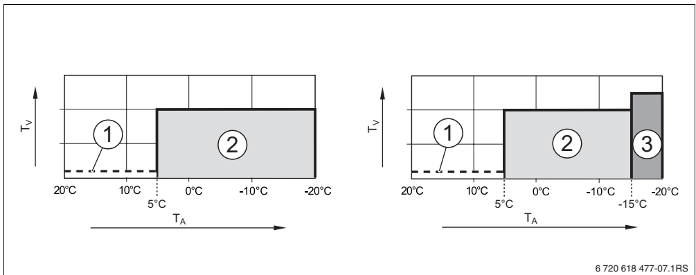
Bild 8 Auswirkung des Parameters „Ab welcher Außentemperatur soll die Absenkung unterbrochen werden?“. Links: Parameter ist auf „Aus“ gestellt (Grundeinstellung). Rechts: Parameter ist auf -15 °C eingestellt
