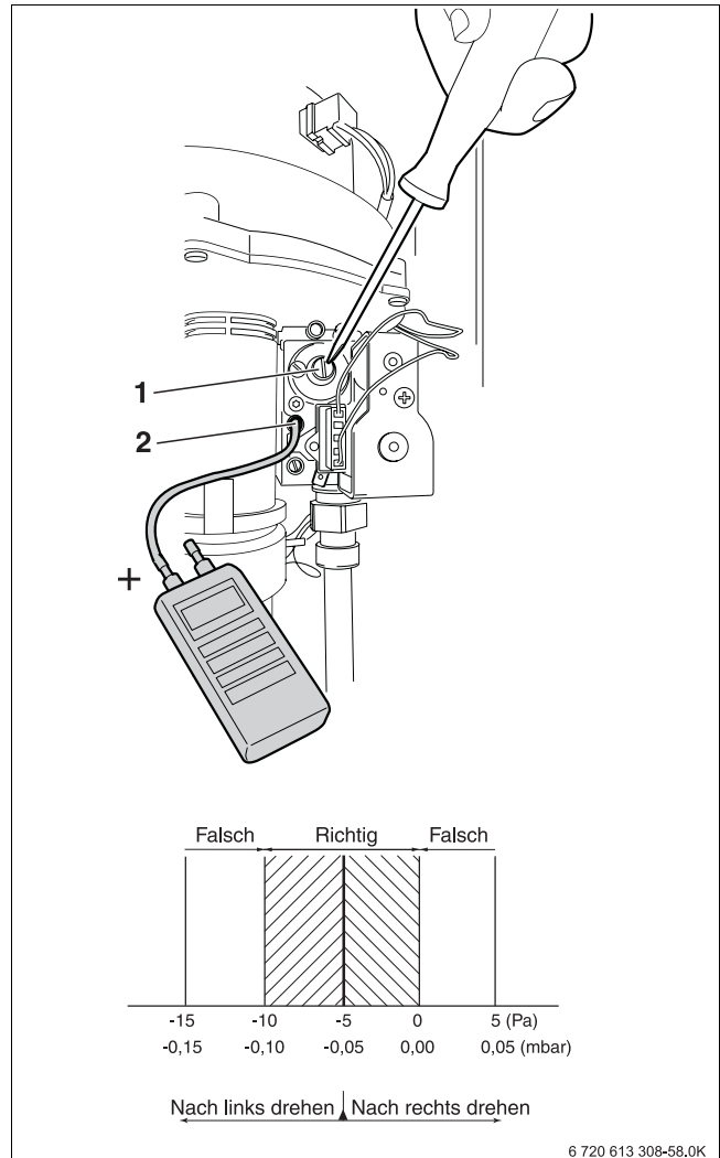
Bild 66 Gas-Luft-Verhältnis einstellen
