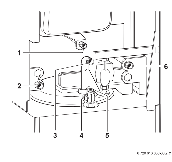
Bild 36 Anschlusssituation GB152-16/24T 83/120/150
