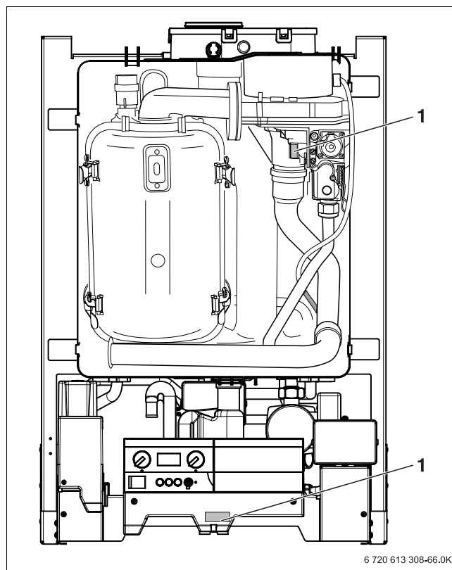
Bild 86 Gasarten-Aufkleber
