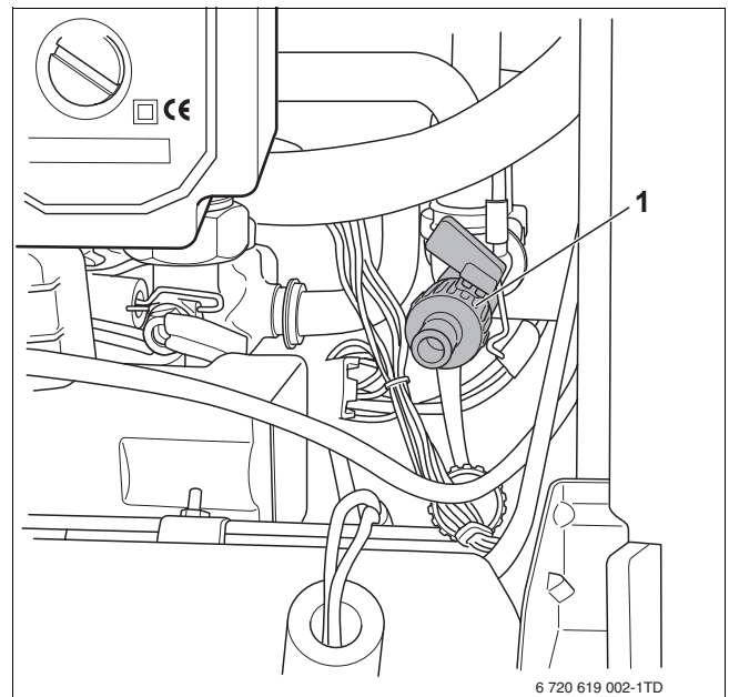
Bild 59 Kesselfüll- und Entleerhahn im Heizkessel
