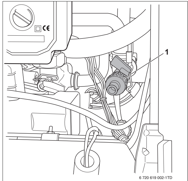
Bild 43 Kesselfüll- und Entleerhahn
