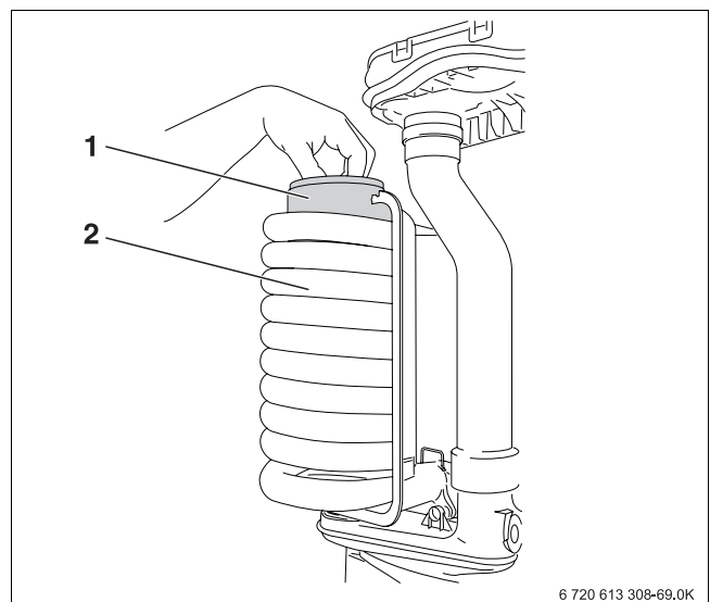
Bild 77 Abgas-Umlenkopf abnehmen
