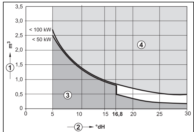
Bild 1 Anforderungen an Kessel-Füllwasser für Logamax-Einzelkessel bis 100 kW
