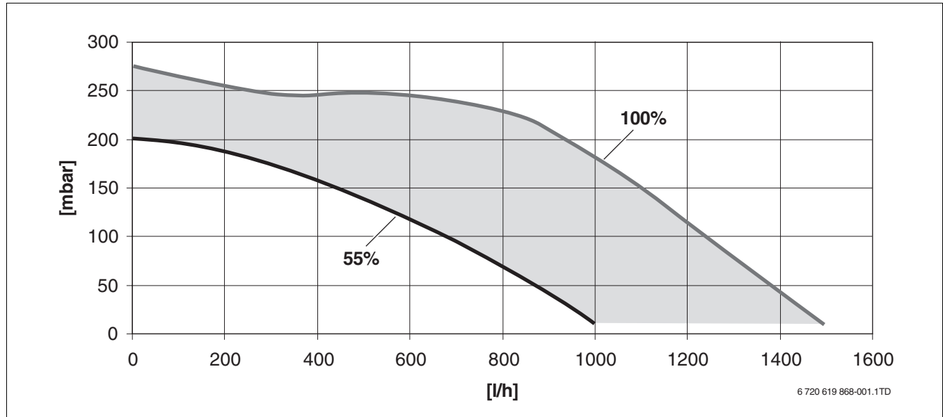
Bild 87 Restförderhöhe für GB152-16/24T mit Hocheffizienzpumpe (mit Bypass 250 mbar)
