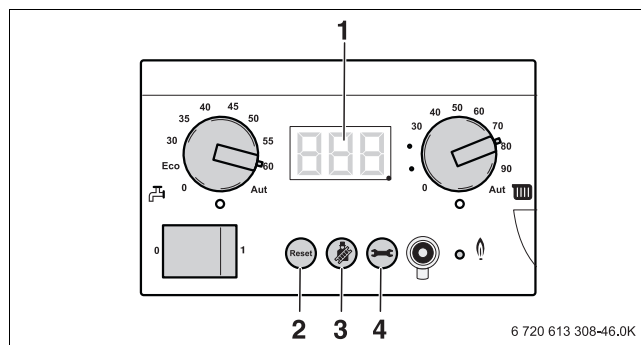
Bild 51 Basiscontroller BC10
