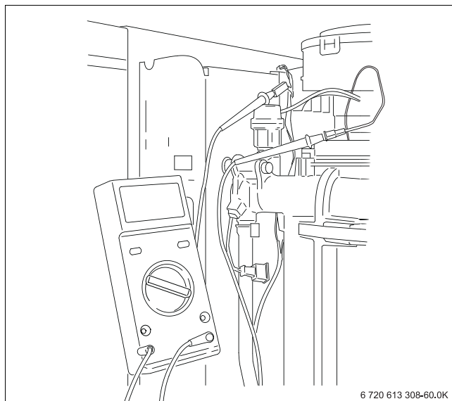
Bild 68 Ionisationsstrom messen
