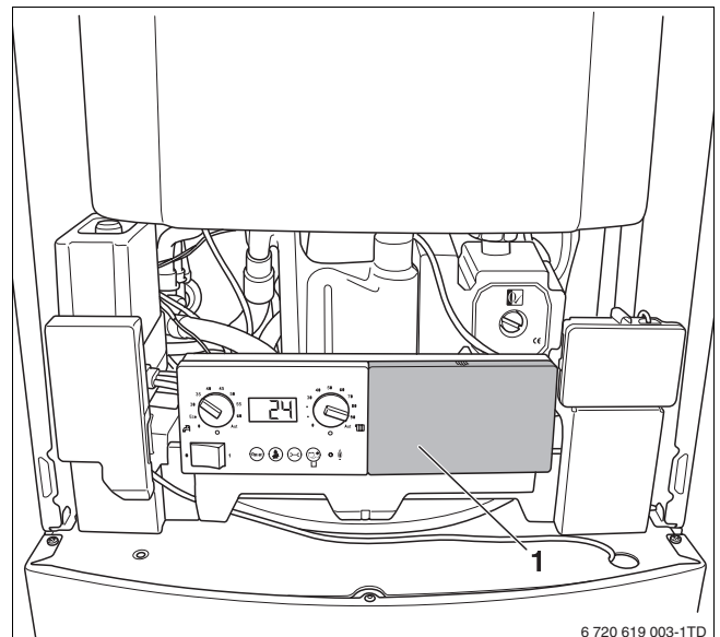
Bild 47 Bedieneinheit montieren
