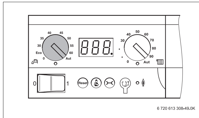
Bild 54 Warmwasser-Sollwert vorgeben
