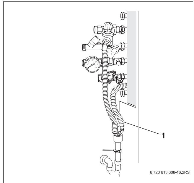
Bild 35 Kondenswasserableitung bei z. B. seitlichem Anschluss-Set (Zubehör)
