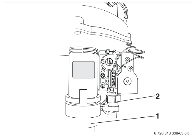
Bild 83 Gasarmatur
