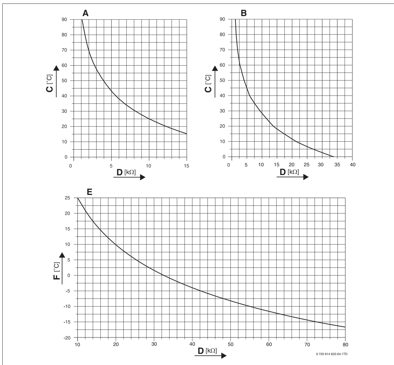
Bild 88 Fühlerkennlinie
