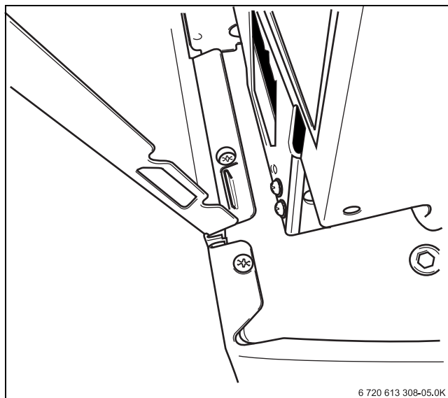
Bild 32 Seitenwände anbringen
