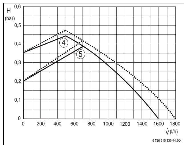
Fig. 56 presiune proporțională
