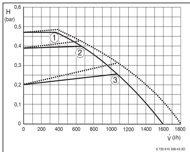
Fig. 55 presiune constantă
