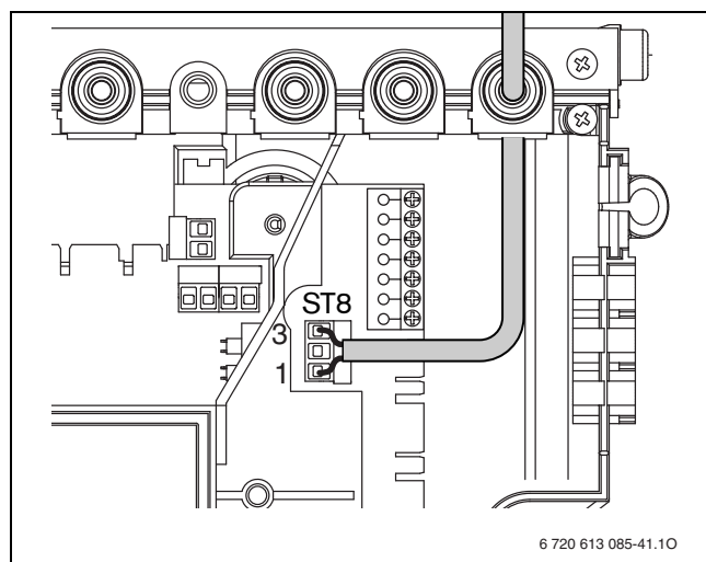
Fig. 33 Racordarea termostatului de boiler
