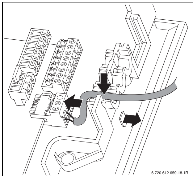
Fig. 32 Racordul senzorului pentru temperatura boilerului (NTC)
