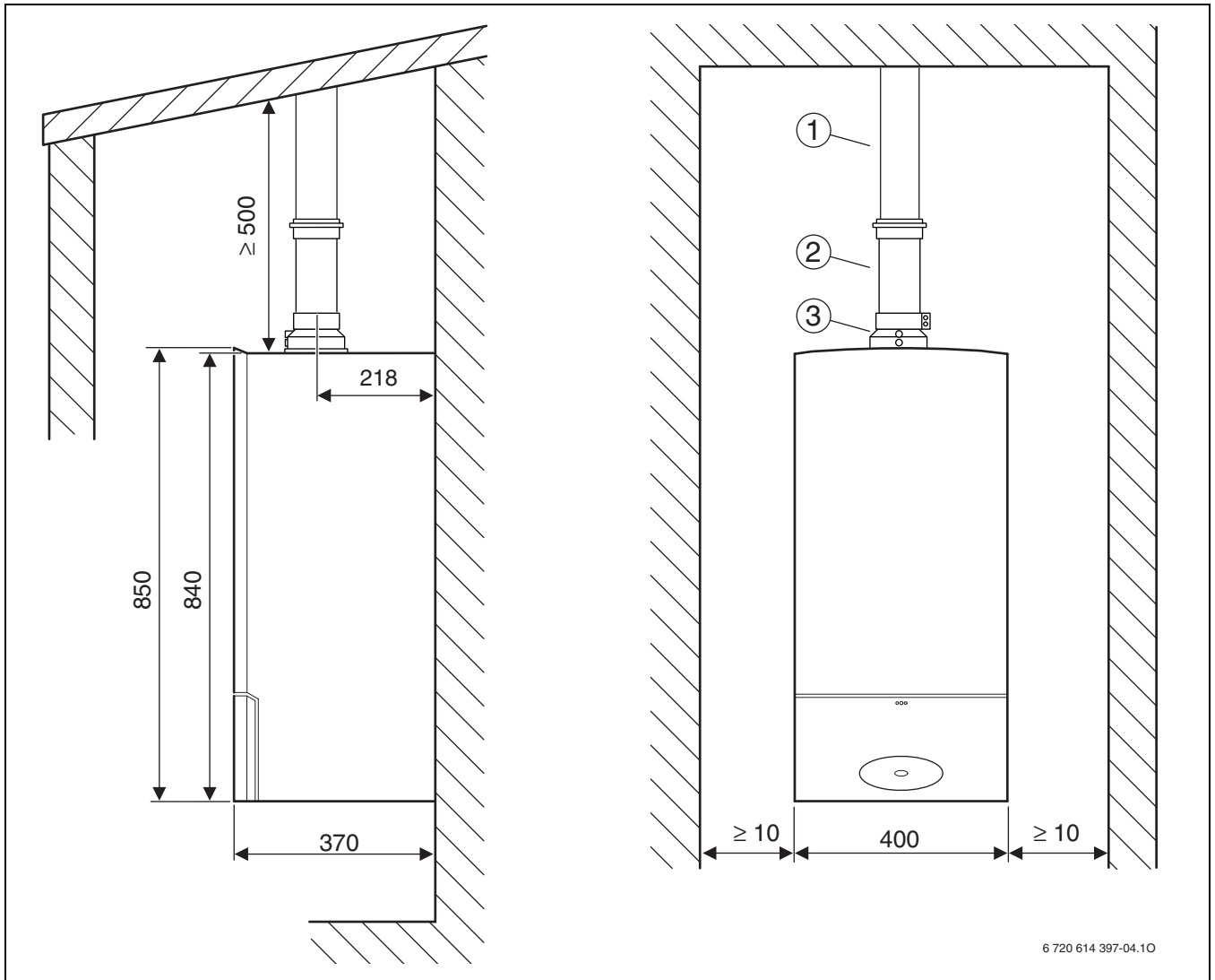
Fig. 8 Acoperiș înclinat
