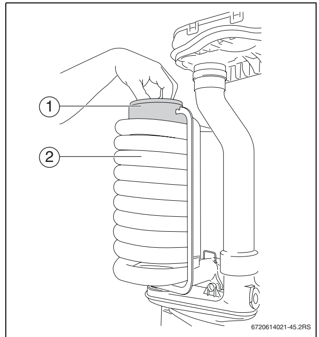
Bild 64 Abgas-Umlenkopf abnehmen
