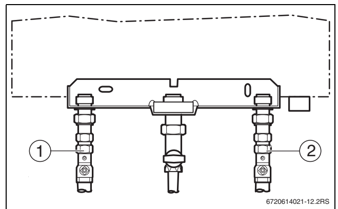
Bild 9 Rohranschlüsse Überputzmontage
