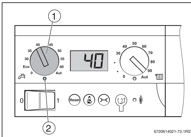
Bild 50 Drehknopf „Warmwasser-Sollwert“
