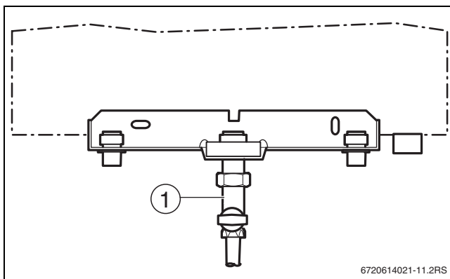
Bild 8 Gasanschluss herstellen
