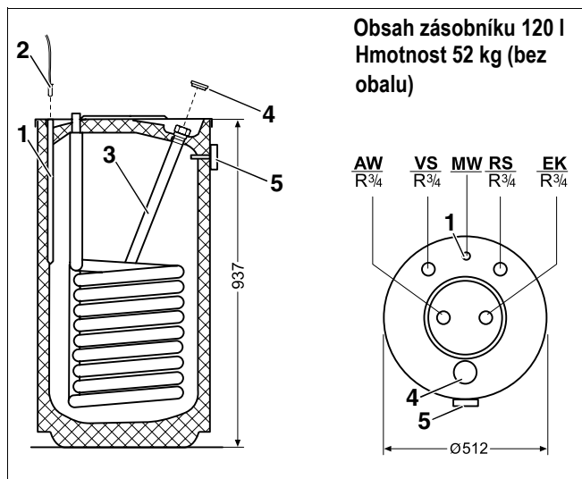
Obr. 1 Přípojky a technická data (rozměry v mm)
