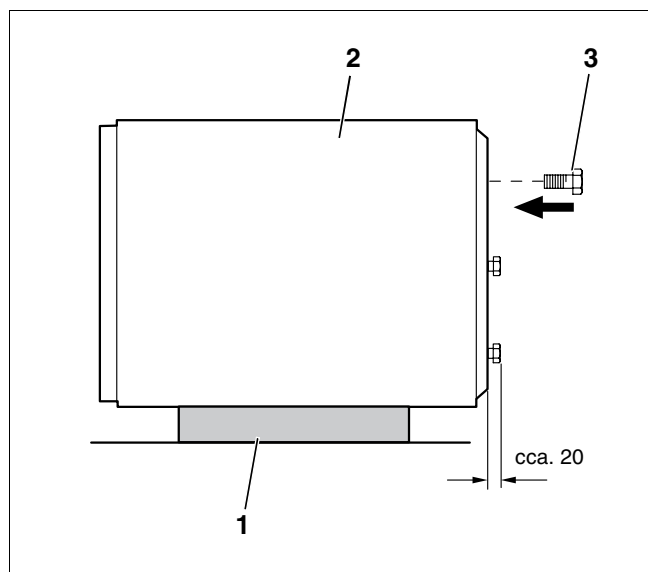
Obr. 3 Zásobník na polštář víka (Princiální zobrazení, míra v mm)
