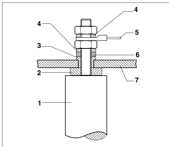
Obr. 7 Instalace hořčíkové anody
