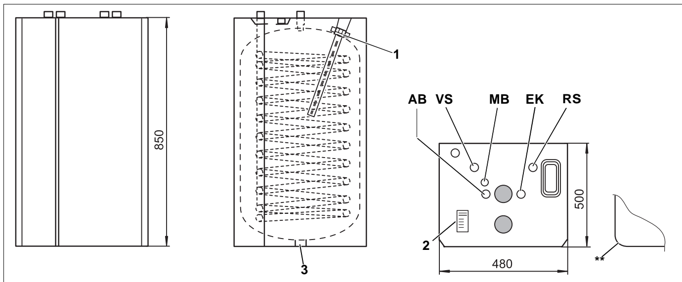
Abb. 1 Abmessungen Logalux HT 110 W/H 110 W
