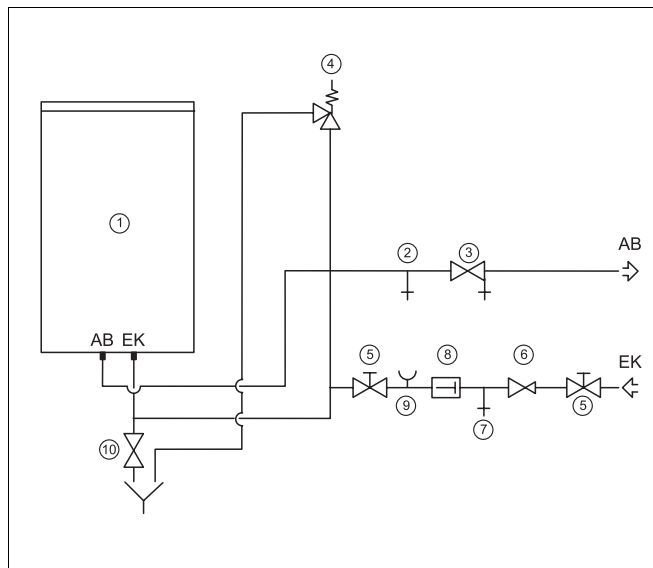
Abb. 9 Installationsschema (Prinzipdarstellung)
