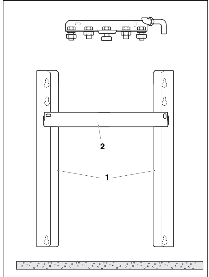
Resim 1 Montaj çerçevesi,
