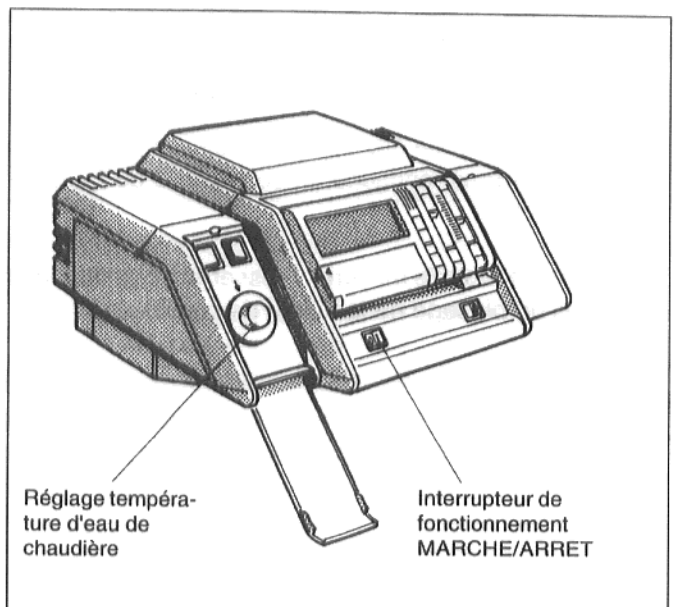
Fig. 27 : système de régulation 4000
