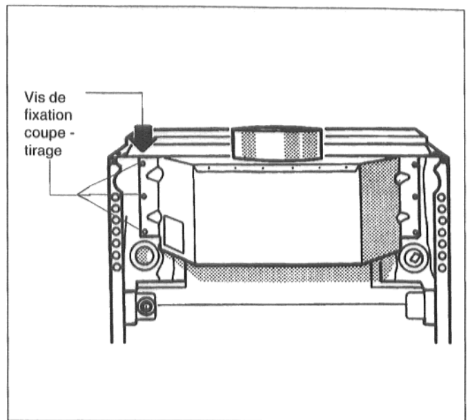
Fig. 5 : montage du coupe-tirage chaudière G 324 XZ
