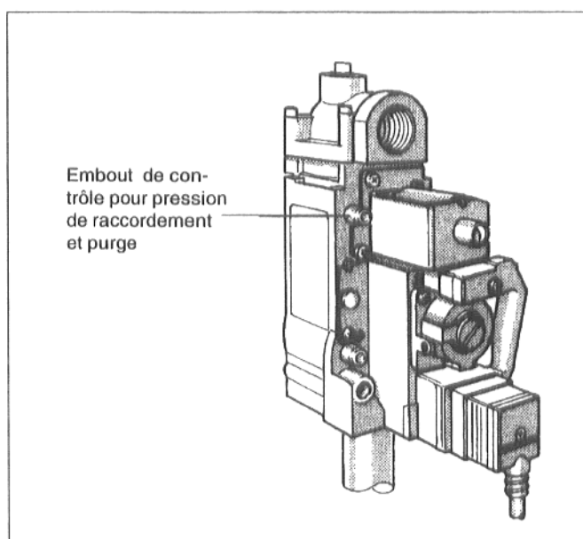
Fig. 30: Bloc de sécurité gaz "Honeywell " VR 4601
