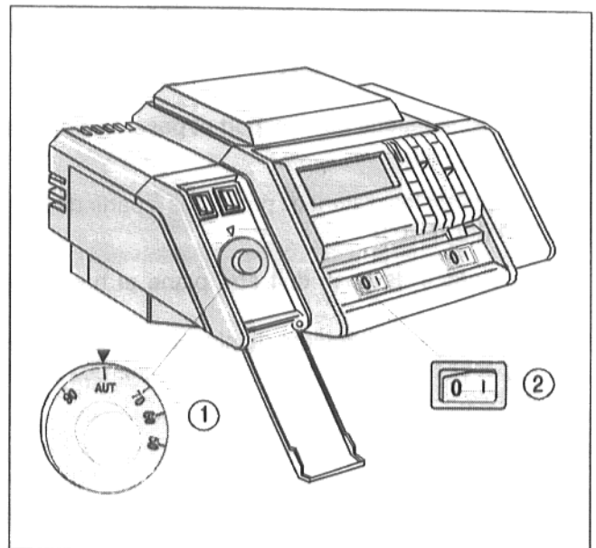
Fig.2 : Système de régulation 4000
