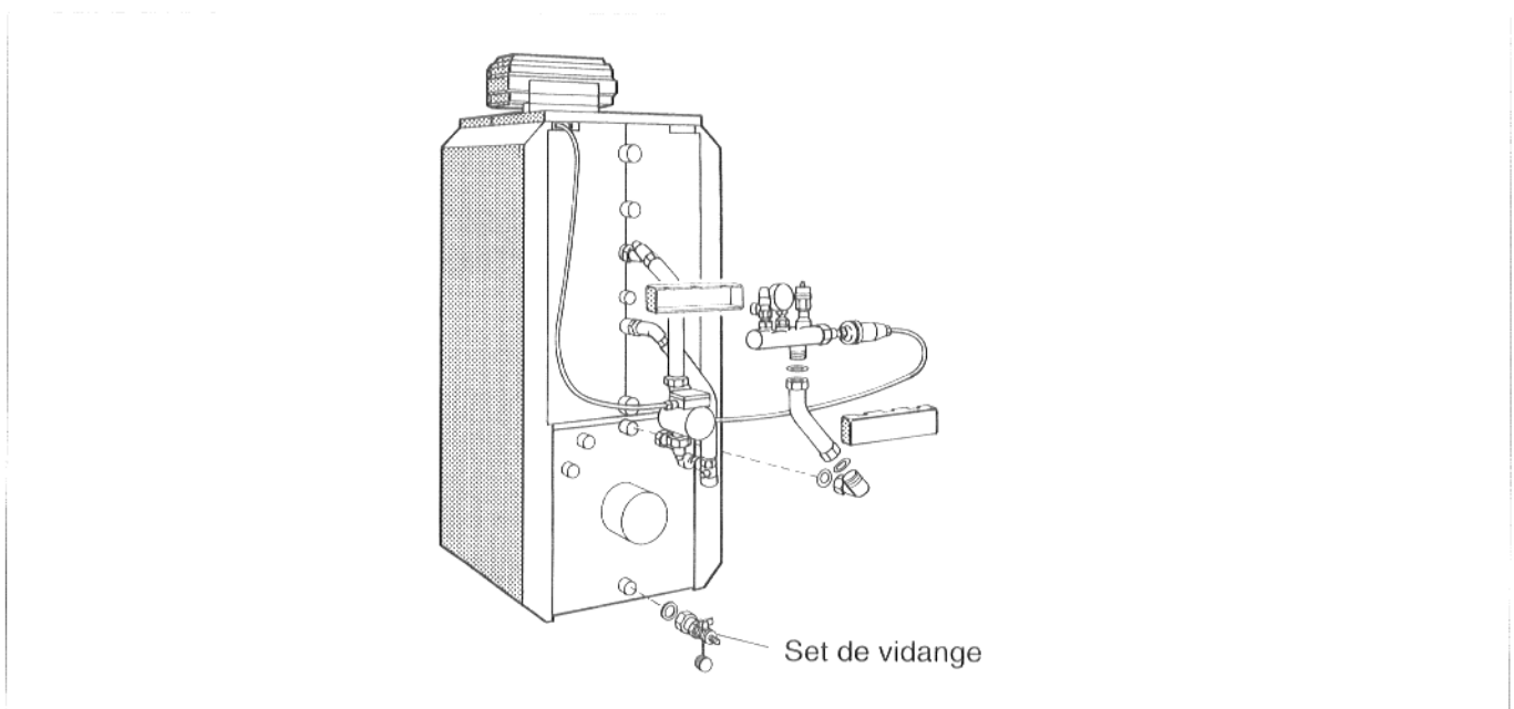
Fig. 6 Set de vidange chaudière pour chaudière S115 T/UT
