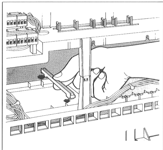
Abb. 3: Führungsschienen aufstecken
